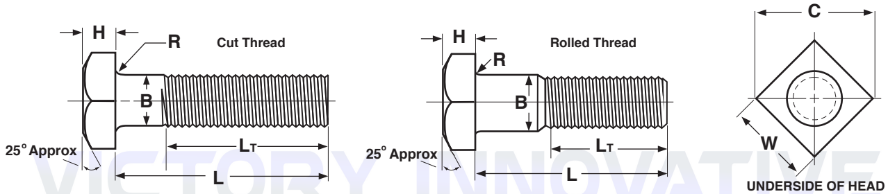
SQUARE BOLTS ASME B18.2.1-2012
